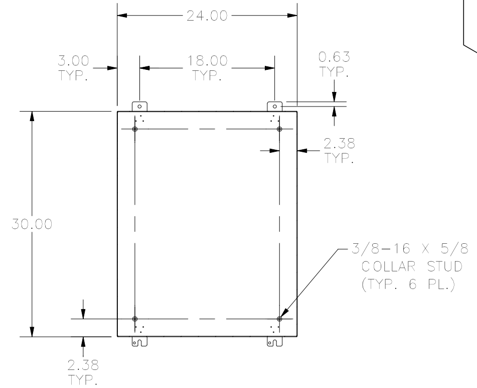
SECTION A-A
