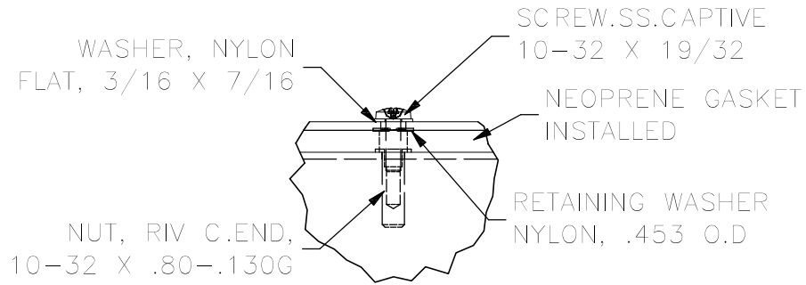
DETAIL D (8 PL.)
