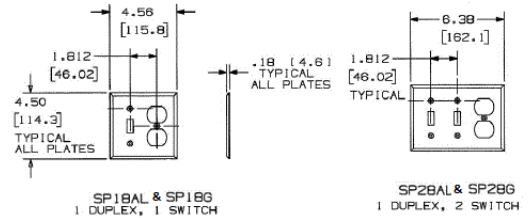
SP18AL & SP18G 1 DUPLEX, 1 SWITCH
