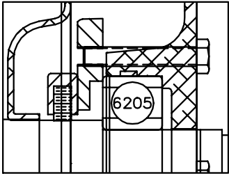
PU END DETAIL
