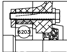
DETAILS OF PU END
