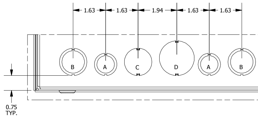
DETAIL B (2 PL.) (K.O. PATTERN)
