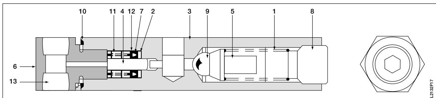
Figure 19, Soupape d'allégement
