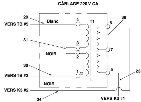
Figure 8, Schéma de câblage (Voir tableau de câblage de la pompe à la page suivante.)
