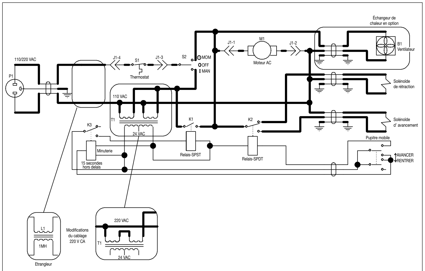
Figure 20, Schéma électrique
