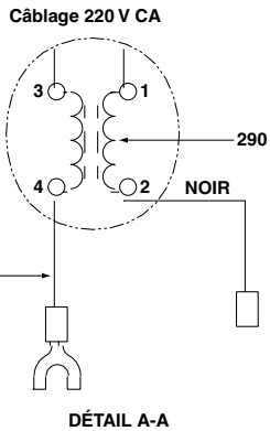
Figure 8, Schéma de câblage (Voir tableau de câblage de la pompe à la page suivante.)
