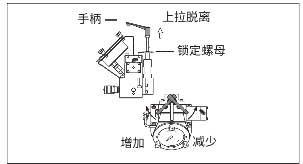
图12- 溢流阀调节
