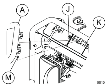
Figura 2-10. Asa de transporte
