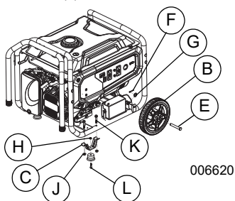
Figura 2-9. Ruedas y patas
