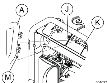
Figure 2-10. Montage de la poignée
