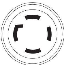
Figura 2-6. Toma de corriente de 120/240 VCA y 30 Amp NEMA L14-30R
