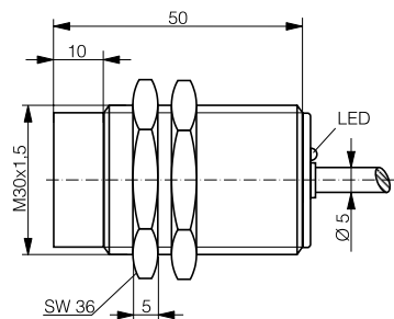
DW-AD-617/618-M30
