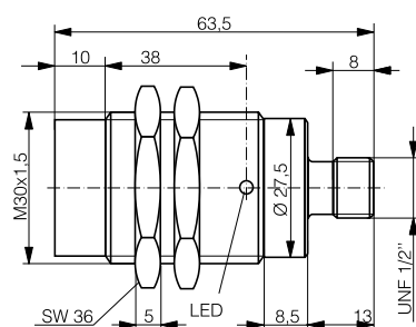
DW-AD-617/618-M30
