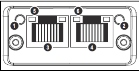
Abb. 1: IMpnio2 interface module, front view (socket)
