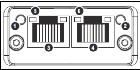
Abb. 1: Schnittstellenmodul IMpno2, Frontansicht (Buchse)
