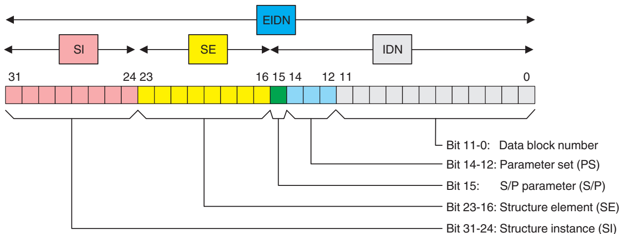
Fig. 2-6 sercos parameter model
