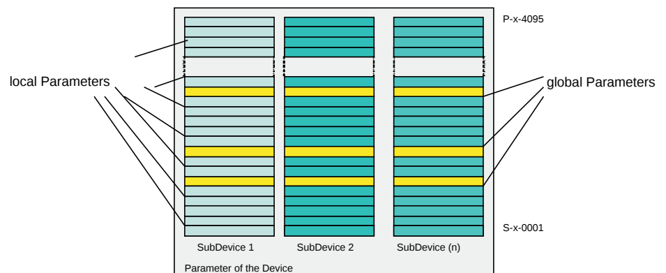
Fig. 2-9 Parameter addressing of global and local parameters
