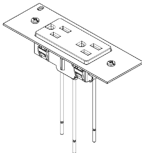
Prise câblée avec sa plaque N° catalogue série PWFB10MPxxxx PWFBMPDR15 illustrée à titre d'exemple
