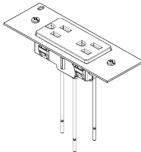
Tomacorriente pre-cableado con placa frontal Catálogo núm. serie PWFB10MPxxx Ejemplo de PWFBMPDR15 mostrado
