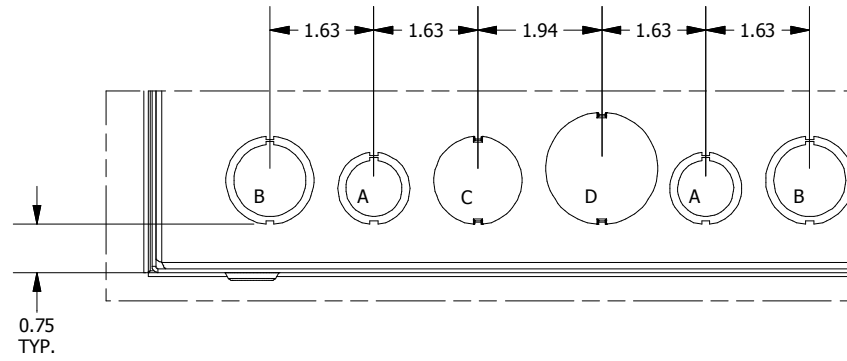
DETAIL B (5 PL.) (K.O. PATTERN)
