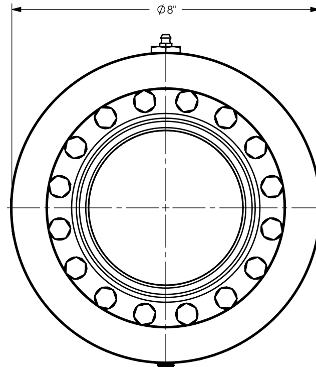
SECTION A-A
