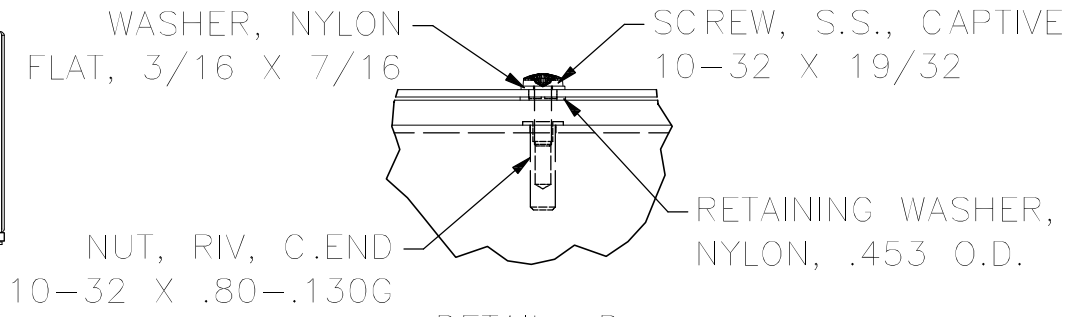
DETAIL D (12 PL.)
